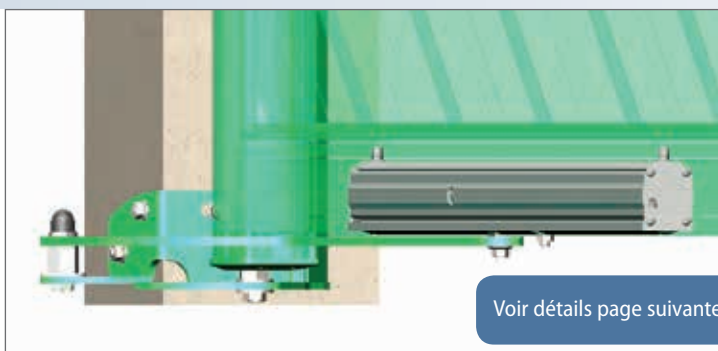
Kit MOTORISATION INTÉGRÉE DANS LA TRAVERSE BASSE (discrétion assurée) Moteur à bras, autobloquant, pour portail 2 vantaux
