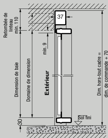
Coupe verticale
